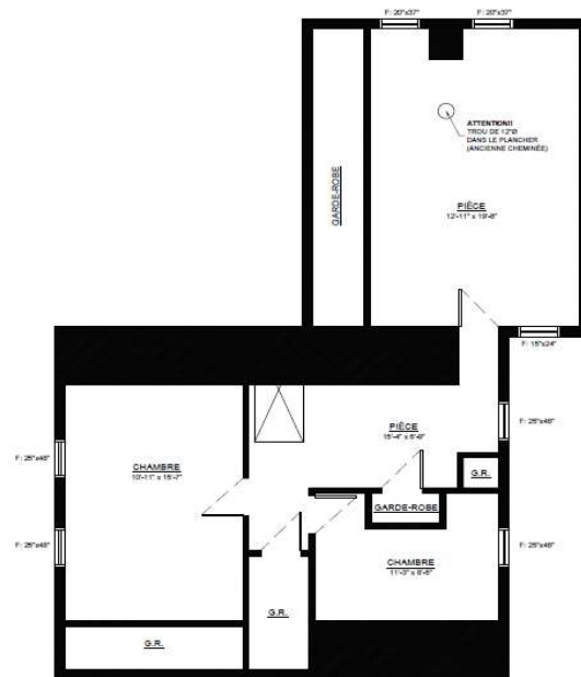
PLAN DU 2 e ÉTAGE
